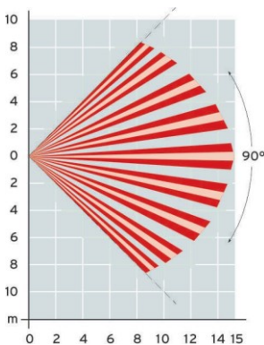
Erfassungsbereich Draufsicht
